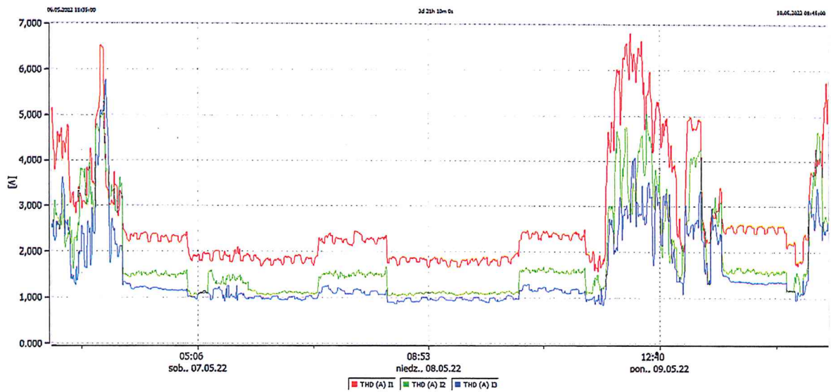
Wykres 4. THDI
