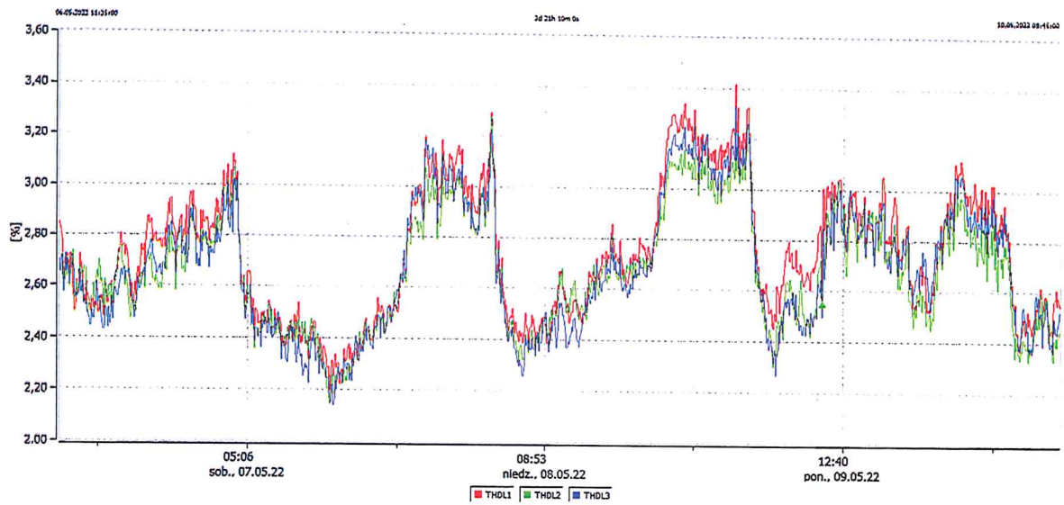
Wykres 3. THDU
